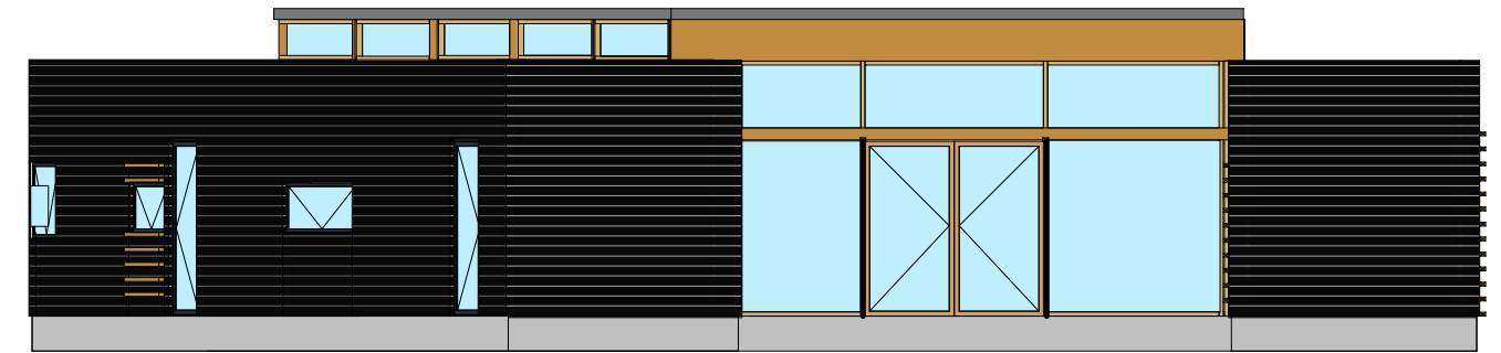
4 "Øst" 1 : 100
